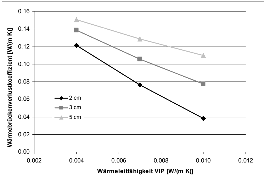
Bild 13 Linienförmige Wärmebrückenverlustkoeffizienten für die Dämmung der Dachterrasse (y-Achse) in Abhängigkeit von der Wärmeleitfähigkeit (x-Achse) und der Dicke des VIP
