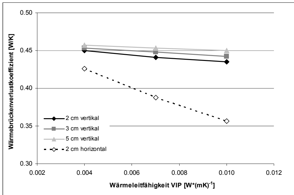
Bild 5 Punktförmige Wärmebrückenverlustkoeffizienten (y-Achse) für die Aussparung Regenfallrohr in Abhängigkeit von der Wärmeleitfähigkeit (x-Achse) und der Dicke des VIP.
