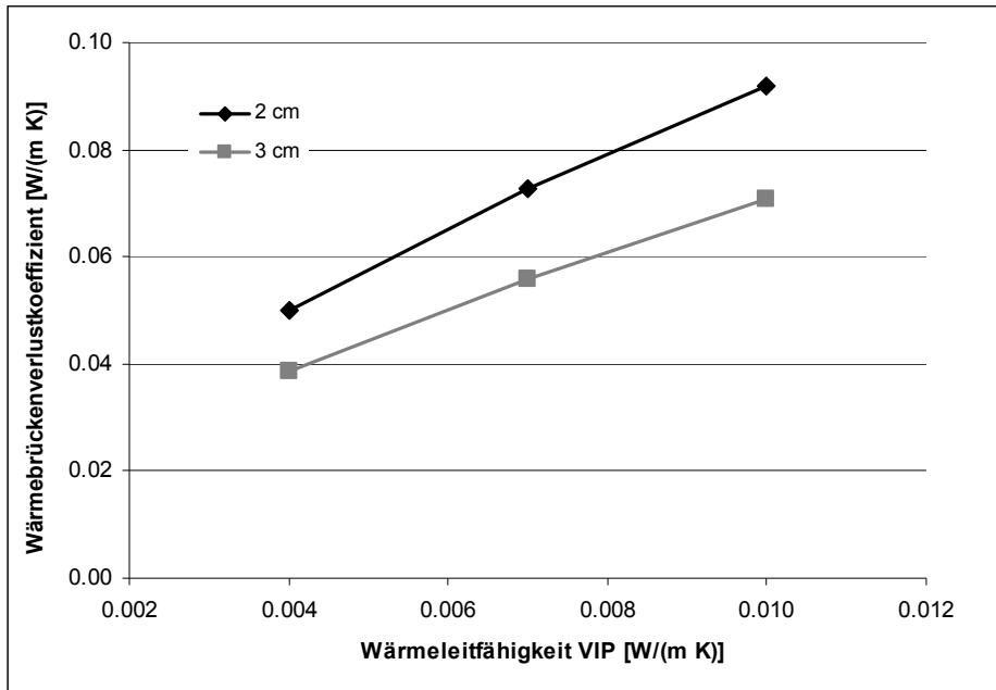
Bild 8 Linienförmige Wärmebrückenverlustkoeffizienten für die Rahmenverbreiterung (y-Achse) in Abhängigkeit von der Wärmeleitfähigkeit (x-Achse) und der Dicke des VIP
