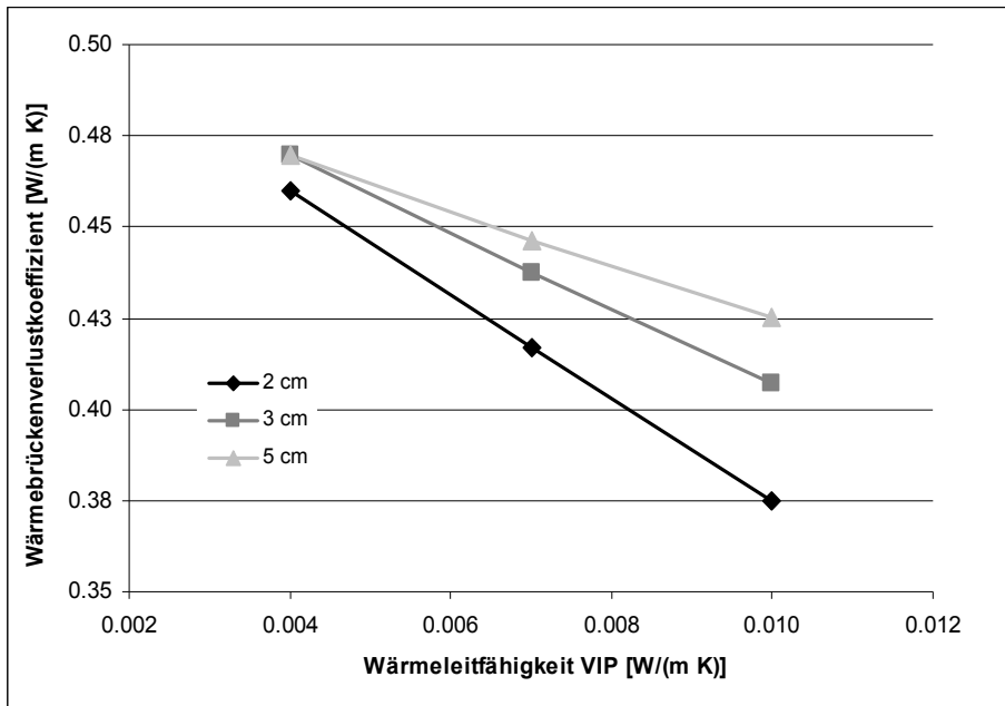
Bild 10 Linienförmige Wärmebrückenverlustkoeffizienten für die Decke gegen unbeheizt (y-Achse) in Abhängigkeit von der Wärmeleitfähigkeit (x-Achse) und der Dicke des VIP
